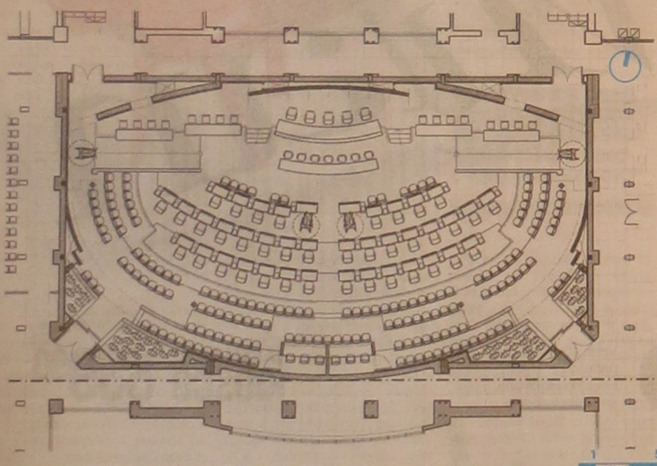
Planta general. El espacio rectangular tipo caja dio lugar a una planta casi oval.
